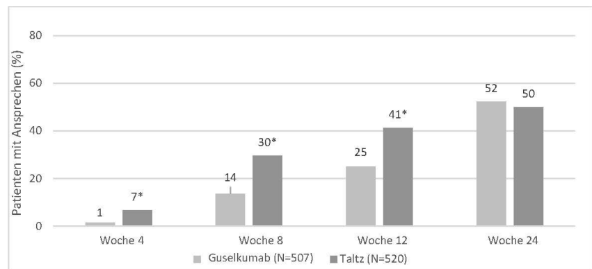
Abbildung 2: PASI 100 in Woche 4, 8, 12 und 24; NRI
